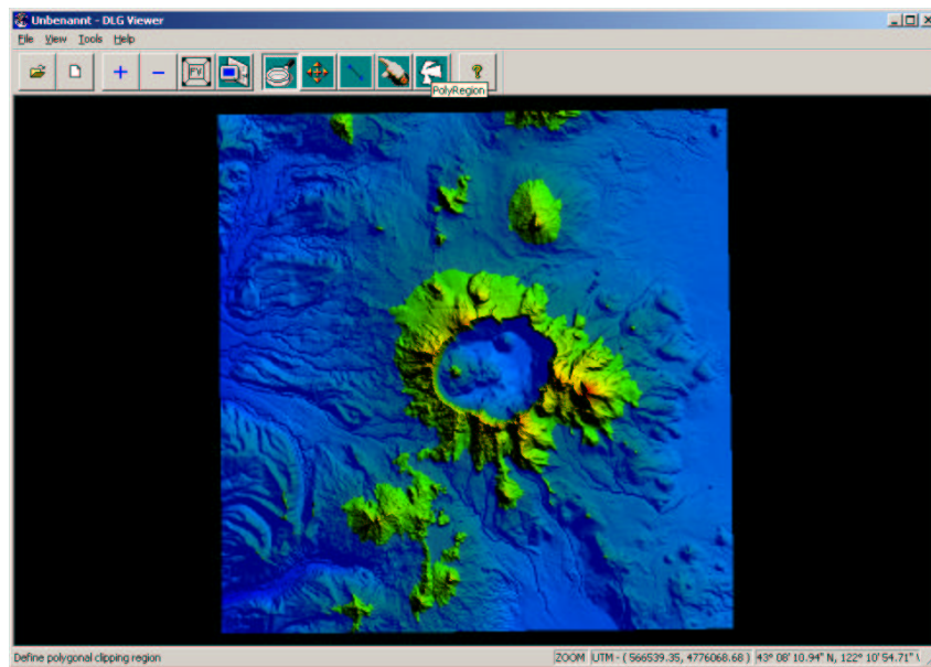
Abbildung 7.3.: Überflutungssimulation „Crater Lake“ Pegelhöhe bei 1900 Metern mit dlgv32
